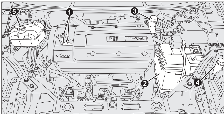
fig. 2a - versione 1.4 Turbo Multi Air
