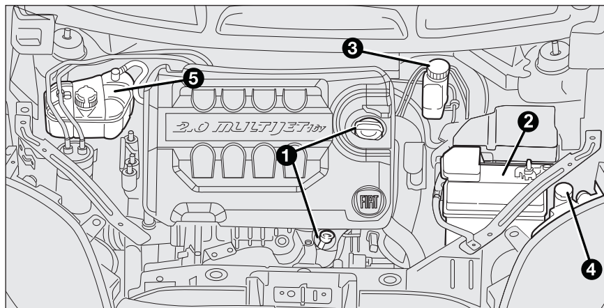
fig. 5a - versione 2.0 Multijet
