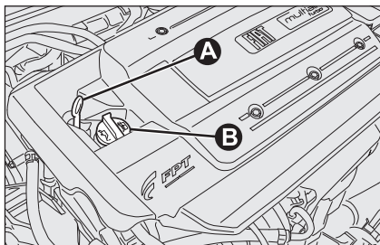
fig. 7a - versione 1.4 Turbo Multi Air
