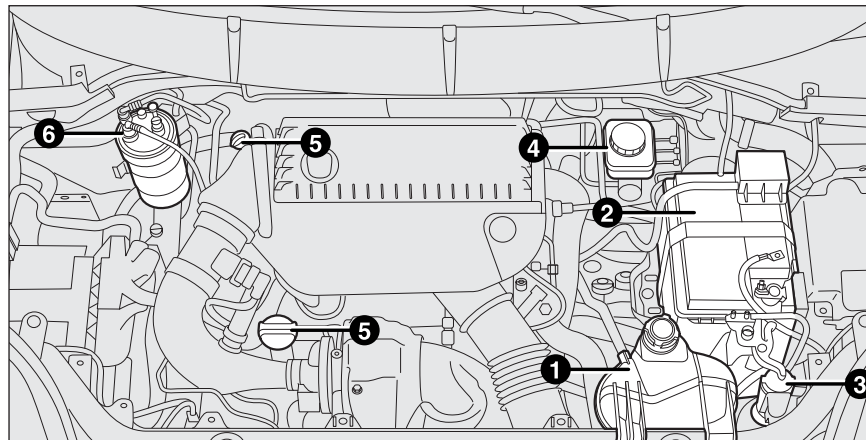
fig. 2a - Versione I.3 Multijet (EURO 5)
