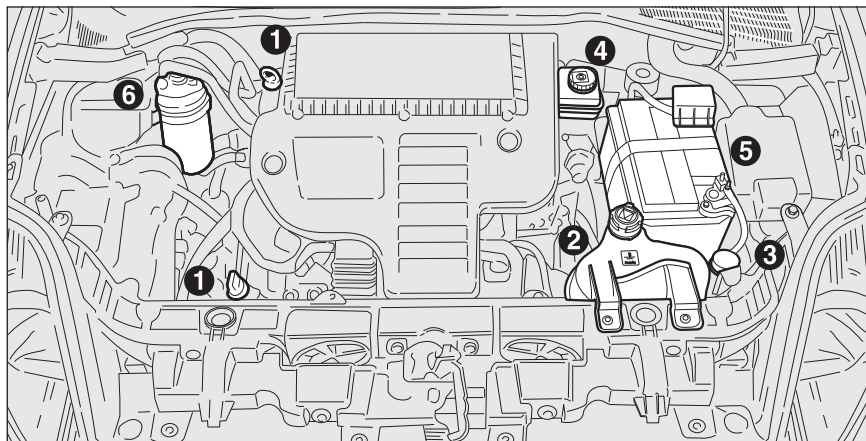
fig. 2 - Versione I.3 Multijet (EURO 4)
