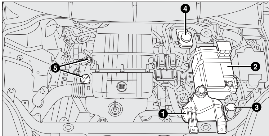
fig. Ia - Versioni 1.2 (Euro 5)
